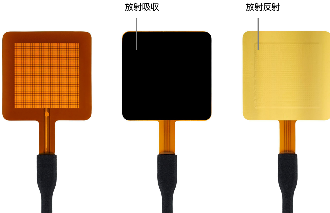
図 0.3 CHF-FHF05-50X50熱流センサ(Mサイズ)(左から、ステッカー無し、BLK-50X50「黒」ステッカー付、GLD-50X50「金」ステッカー付)
