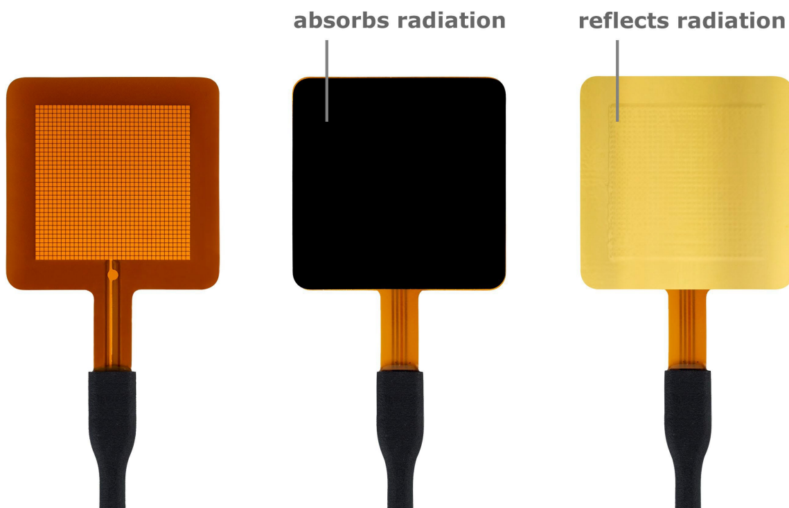
図 7.3.1 CHF-FHF05-50X50(Mサイズ)熱流センサに「黒」「金」ステッカーを貼った状態
