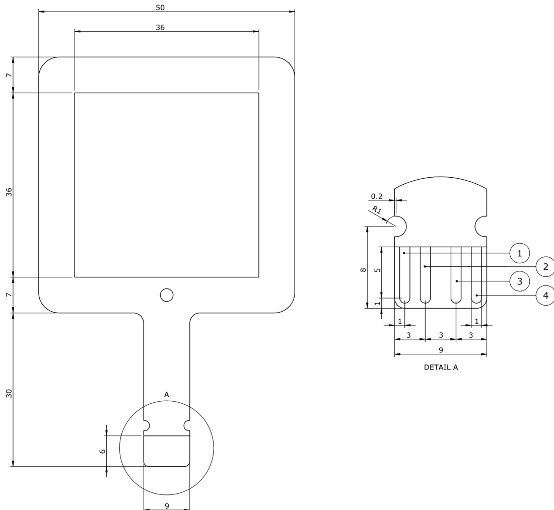
図 7.2.1 CHF-FHF05-50X50(Mサイズ)薄膜センサ:上図DETAIL Aはすべての CHF-FHF05 シリーズで共通です。(寸法は \times 10^{-3} m )
