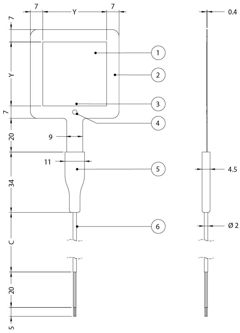
図 3.2.2 CHF-FHF05 10X10(SSサイズ)、50X50(Mサイズ)、85X85モデル(Lサイズ)。Y = 8, 36, 70( \times 10^{-3} m )
