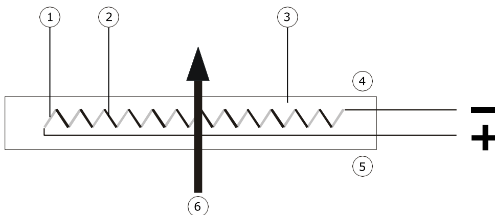
図 2.1 熱流センサの一般的な動作原理。CHF-FHF05に内蔵されているセンサはサーモパイルです。サーモパイルは、2つの金属合金からなる多数の熱電対(①、②)を電氣的に直列に接続したものです。1個の熱電対は、その高温部と低温部の温度差に比例して出力電圧を発生させます。熱電対を直列に並べると、信号が増幅されます。熱流センサでは、高温部と低温部はセンサ面を挟んでそれぞれ反対側に配置されます(④、⑤)。定常状態では、熱流束(⑥)はセンサの温度差とセンサ本体(③)の平均熱伝導率の一次関数となります。サーモパイルは、センサを通過する熱流束に比例した電圧出力を発生させます。センサの正確な感度は、メーカーでの校正によって決定され、センサに付属する製品証明書に記載されています。
