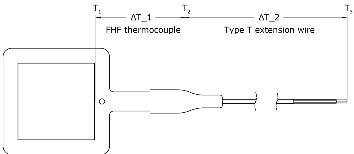
図 7.8.1 CHF-FHF05-50X50(Mサイズ)と熱電対の接合部。不確かさを最小にするために、 \Delta T_1 がゼロに近いことを確認してください。
