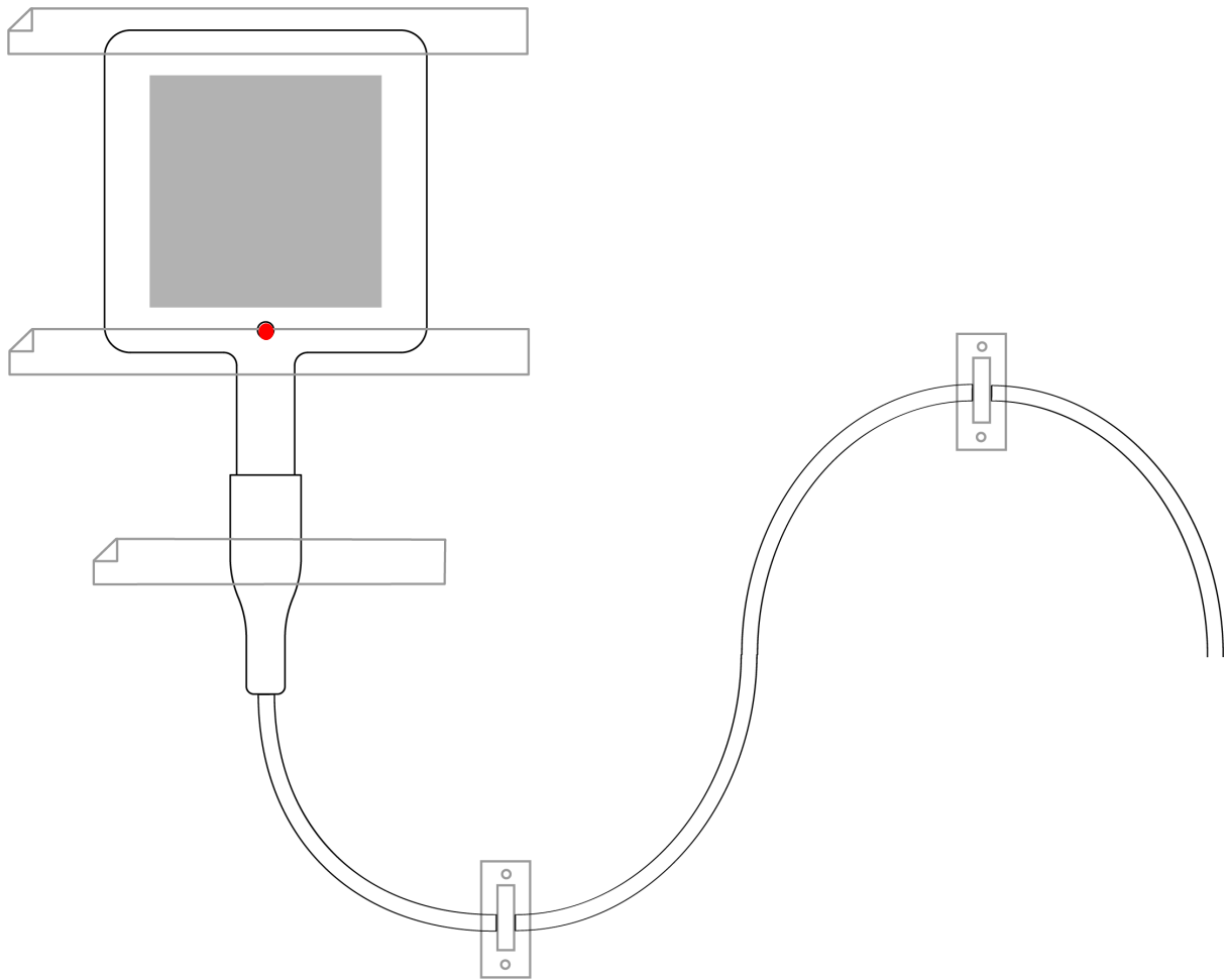
図 5.1.1 CHF-FHF05-50X50モデル(Mサイズ)の設置:センサとコネクタブロックをテープで固定します。両面テープタイプのタイマウントを使用し、ケーブルの負担緩和を行います。表5.1.1に示すように、センサを固定するテープはガード部分に貼るのが好ましく、感部面には貼らないようにします(図5.1.1では灰色の網掛け部分が感部面を示しています)。この図ではドット(上図赤色の部分)がありますが、これは表側であることを示し、裏側は第2章で説明したように、センサを取り付ける対象物に貼り付けられていることを表しています。
