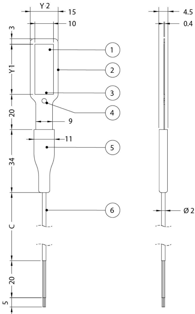
図 3.2.1 CHF-FHF05 15X30モデル(Sサイズ) および 15X85モデル(LGサイズ)。Y1 = 27 または 70、Y2 = 18 または 25 ( \times 10^{-3} m )。
