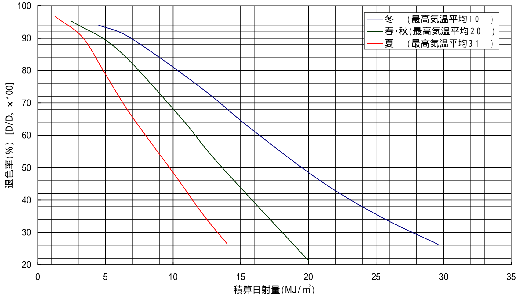
オブリーフ退色曲線(検量線) 「O-1D」 日射量 (東京都実測値)
