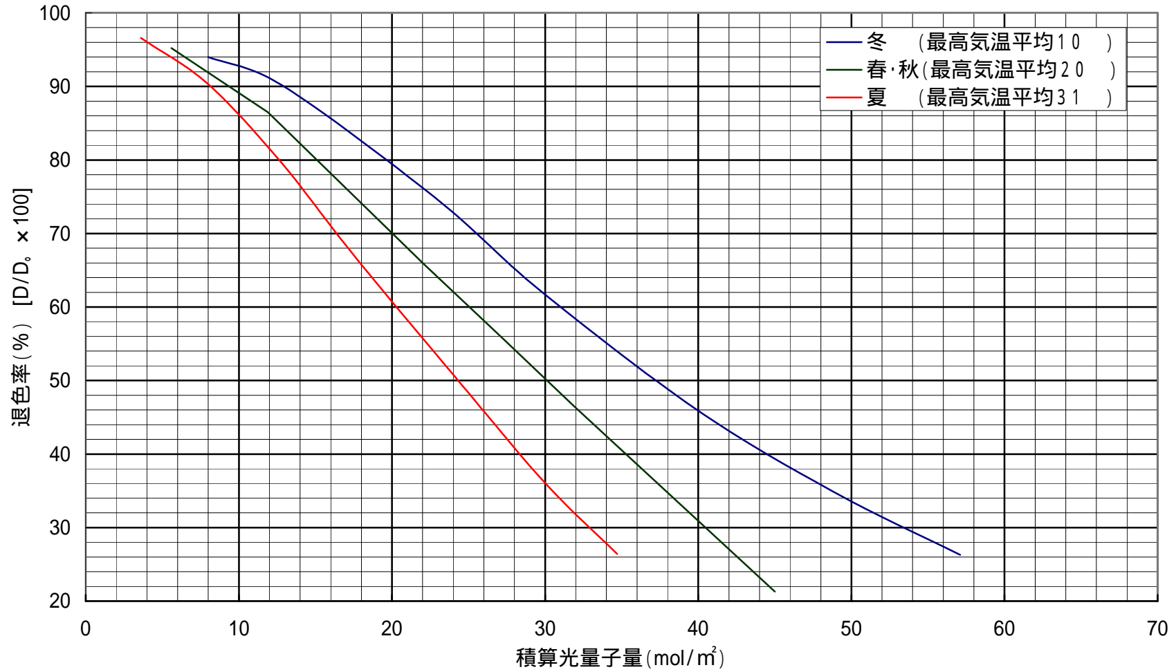
オブリーフ退色曲線(検量線) 「O-1D」 光量子量 (東京都実測値)
