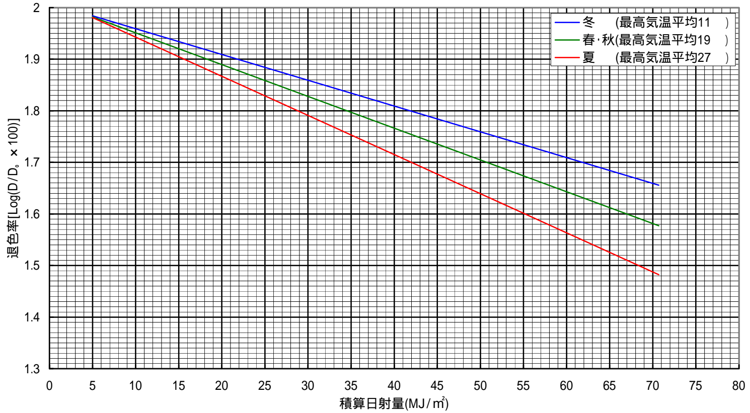
オブリーフ退色曲線(検量線) 「R-3D」 日射量 (千葉市実測値)
