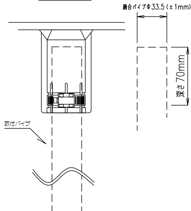
パイプ取付部 矢視図
